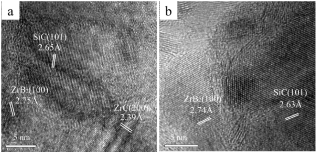
图1 1400 (a)和1600 (b)热处理SiC-ZrB 2 复相陶瓷纤维的微观结构
