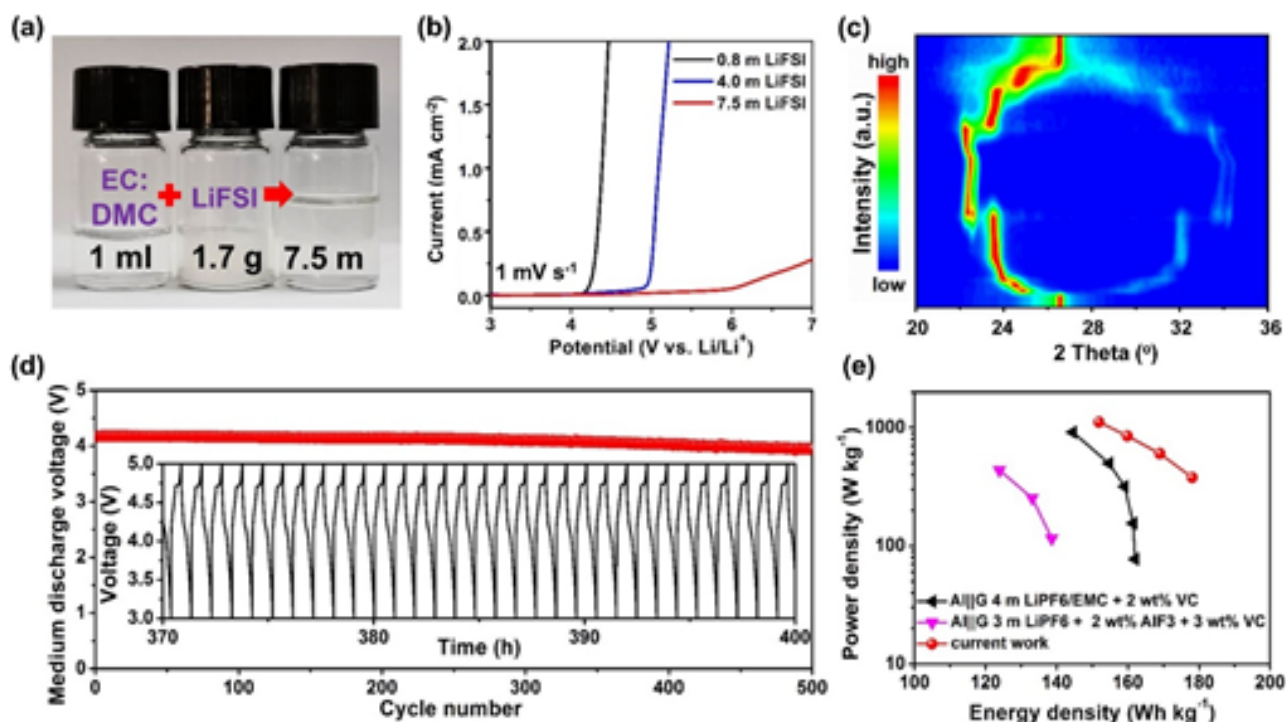
图 (a) 溶剂与电解质盐共溶后获得高浓度电解液的照片；(b) 不同浓度电解液的抗氧化LSV曲线比较；(c) 高浓度电解液体系中，阴离子插层石墨正极的原位XRD表征；(d) 双离子电池长循环过程的放电中压(插图为长循环过程中的充放电曲线)；(e) 已报道双离子电池能量密度比较。
