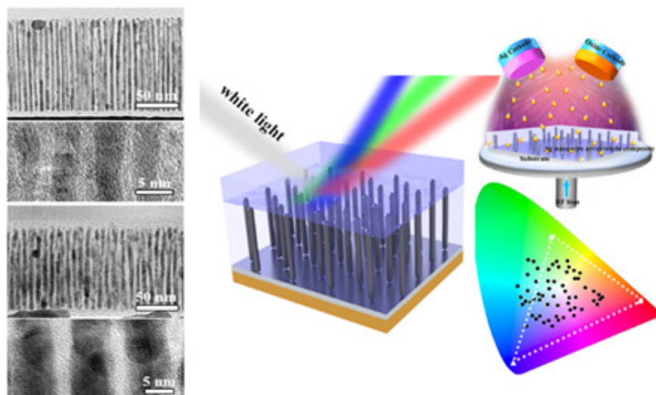
图1.Ag纳米线阵列微结构的精细调控及新型等离激元结构色材料和制备
