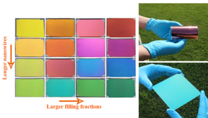
图2.等离激元结构色板和大面积柔性样品
