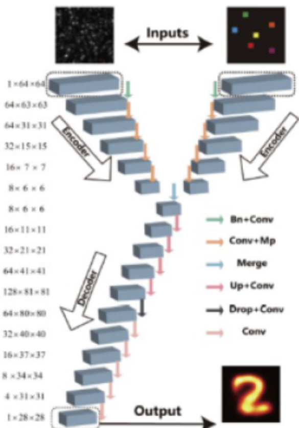
动态解码网络模型 (Y-Net) 及实验结果
