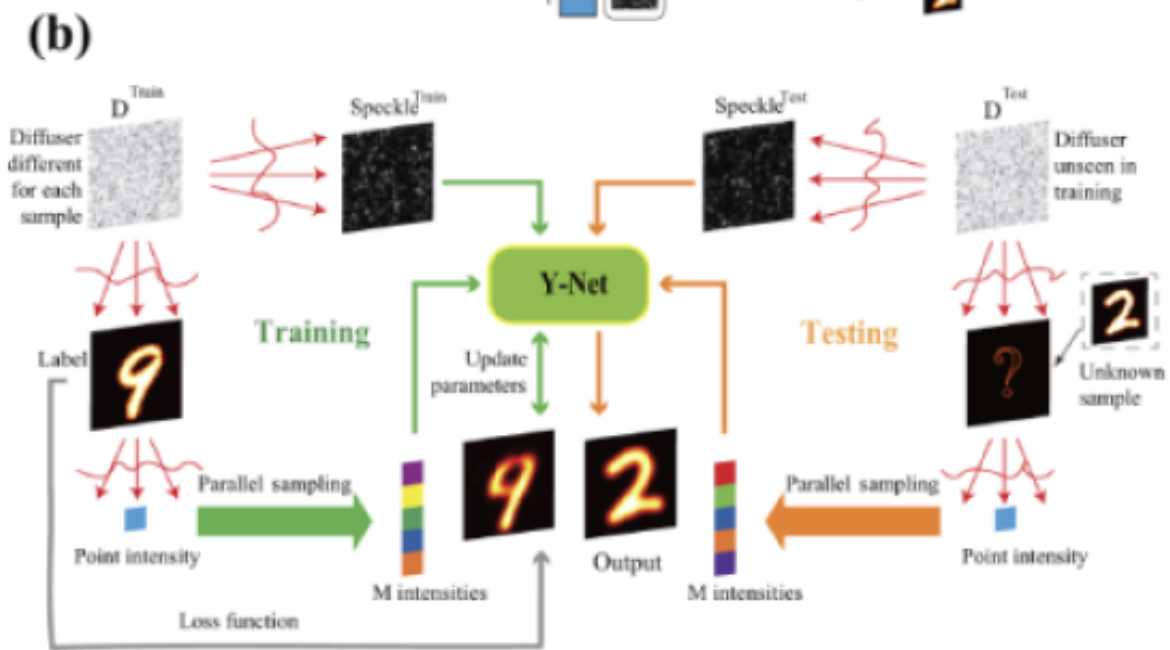
基于深度学习的傅里叶变换关联成像原理 (a) 成像光路 (b) 网络数据流
