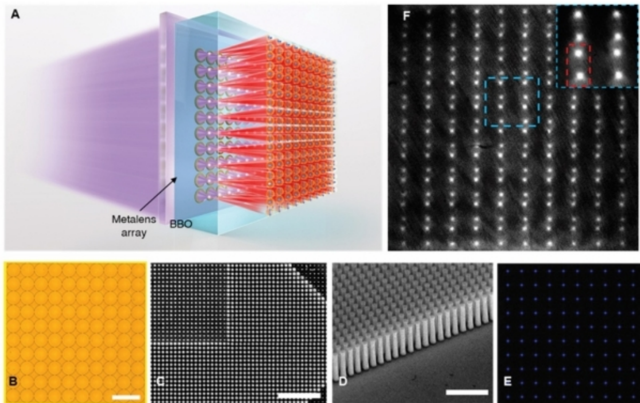
基于超构透镜阵列的量子光源系统
