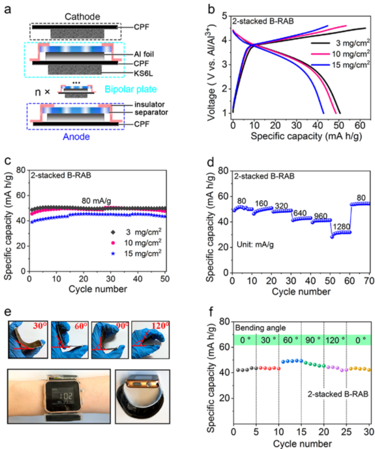
图3 4V双极型可充铝电池电化学性能
