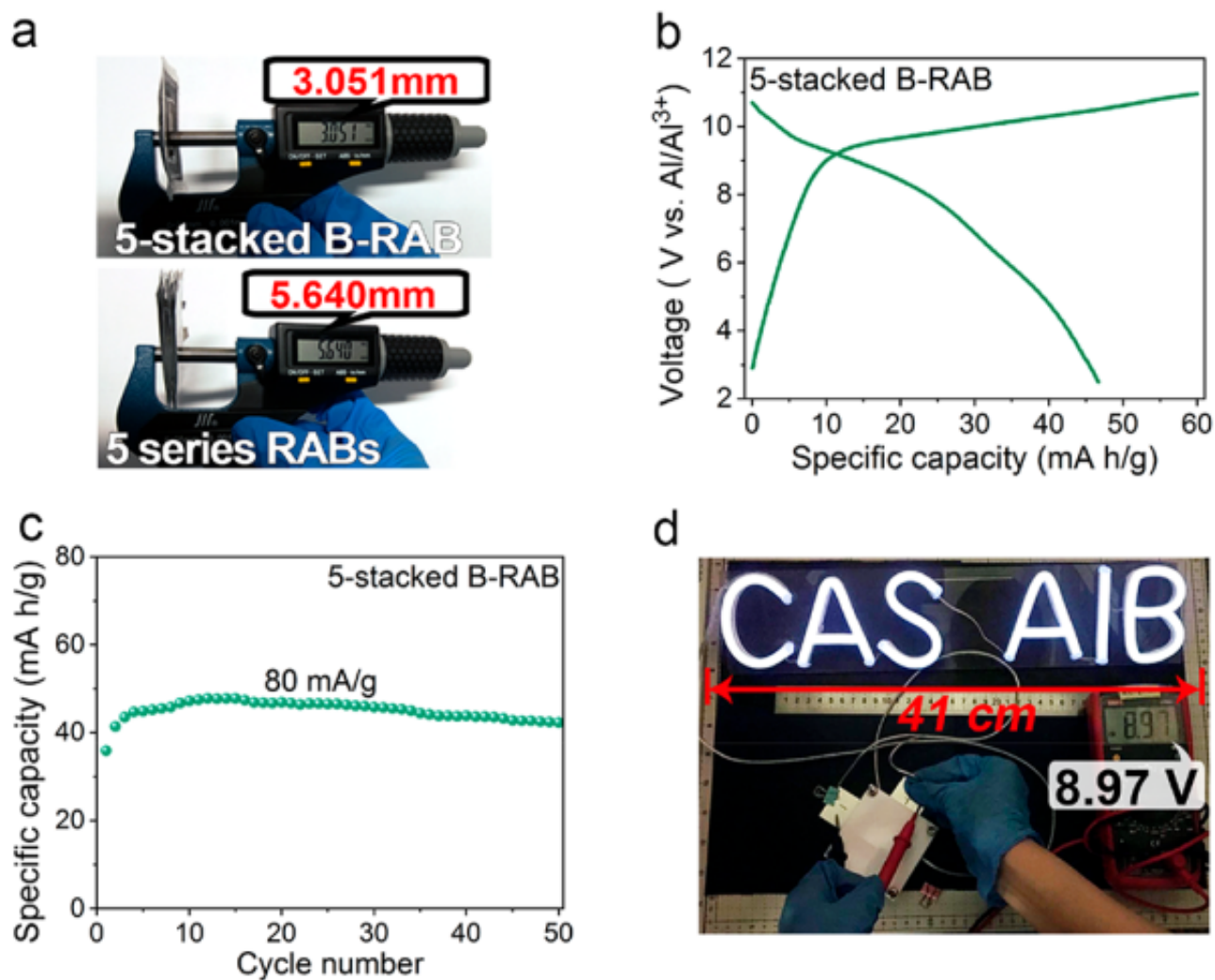
图4 10V双极型可充铝电池电化学性能
