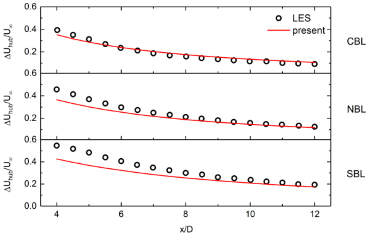
图4 不同大气稳定度下轮毂高度的速度亏损
