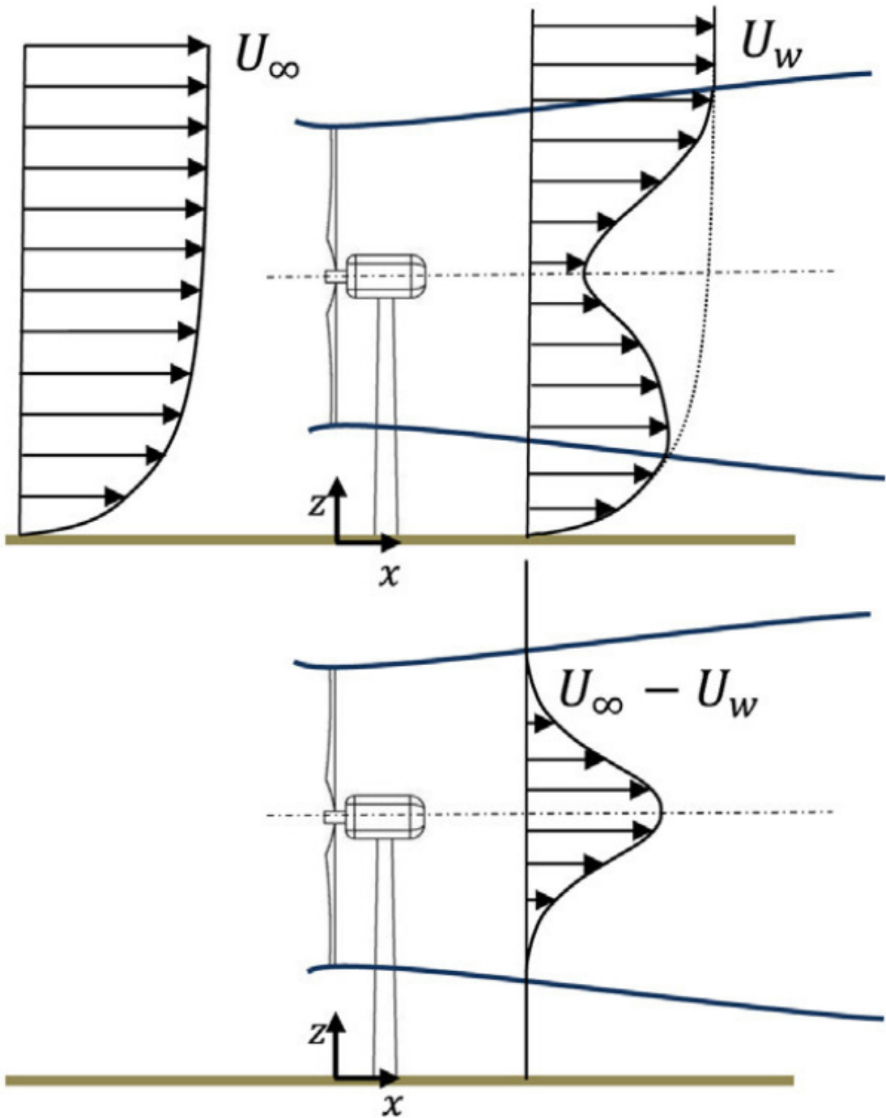
图2 高斯分布形式的速度亏损
