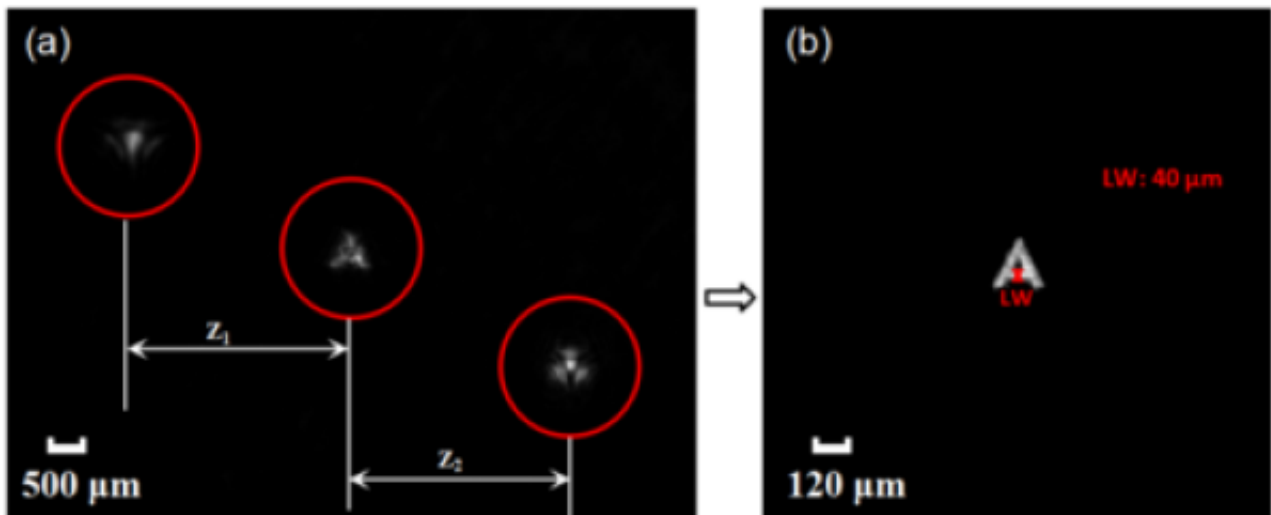
图2 实验结果。(a)CCD记录的单帧衍射场，(b)重构像。
