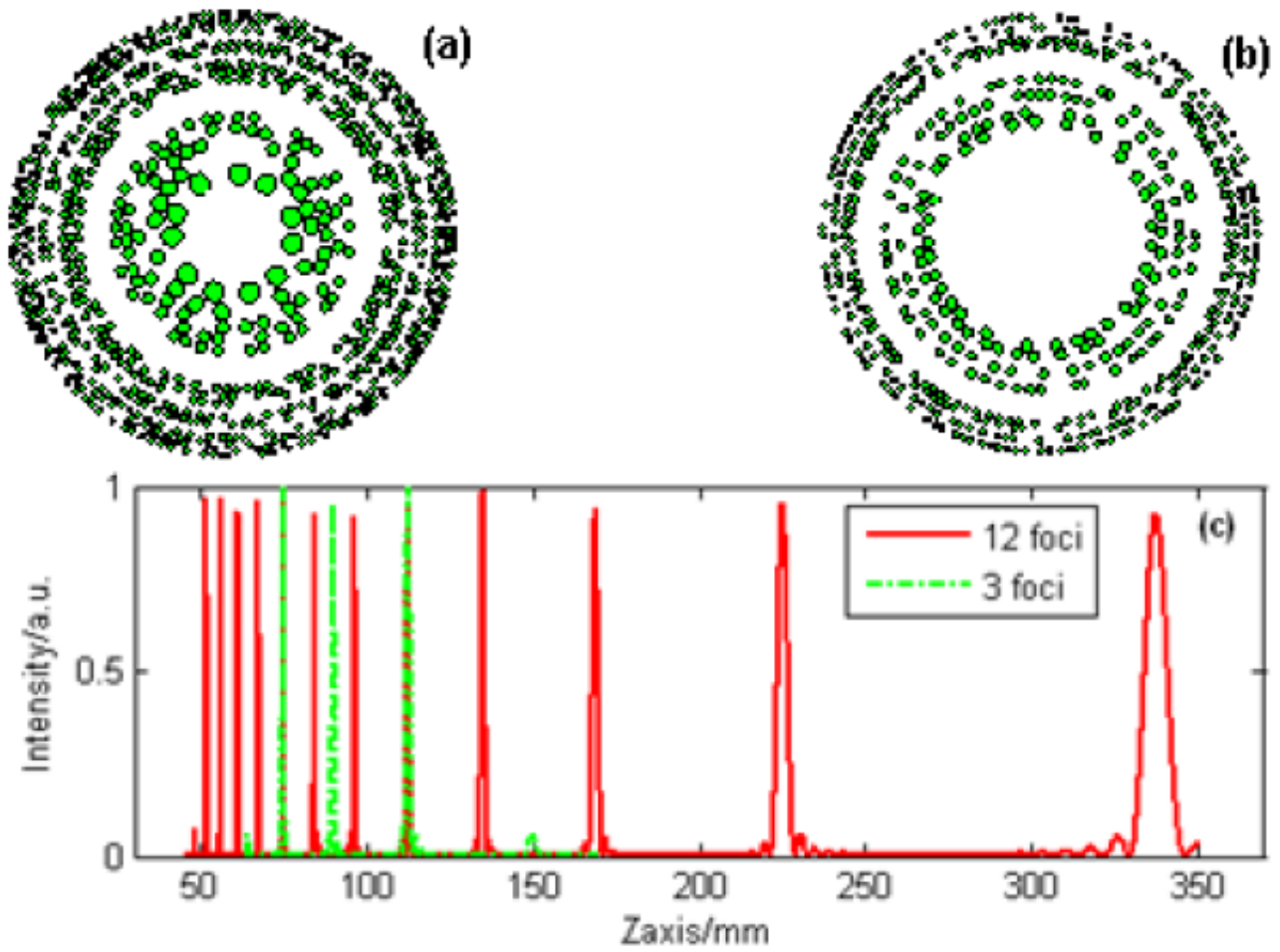
图1 前20环斐波那契光子筛。(a)12焦点，(b)3焦点，(c)轴上光强分布。
