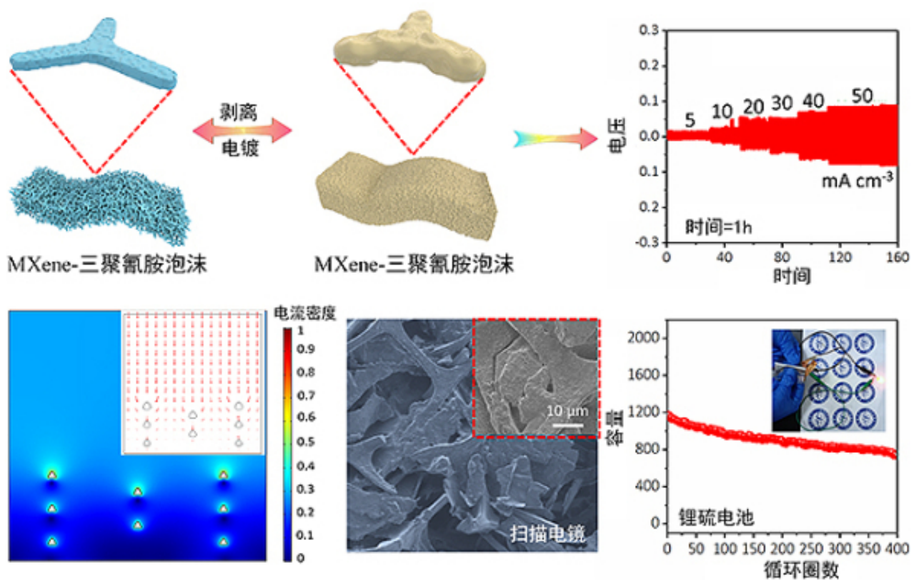
三维MXene-三聚氰胺泡沫用于高电流密度、高容量碱金属电极的原理图
