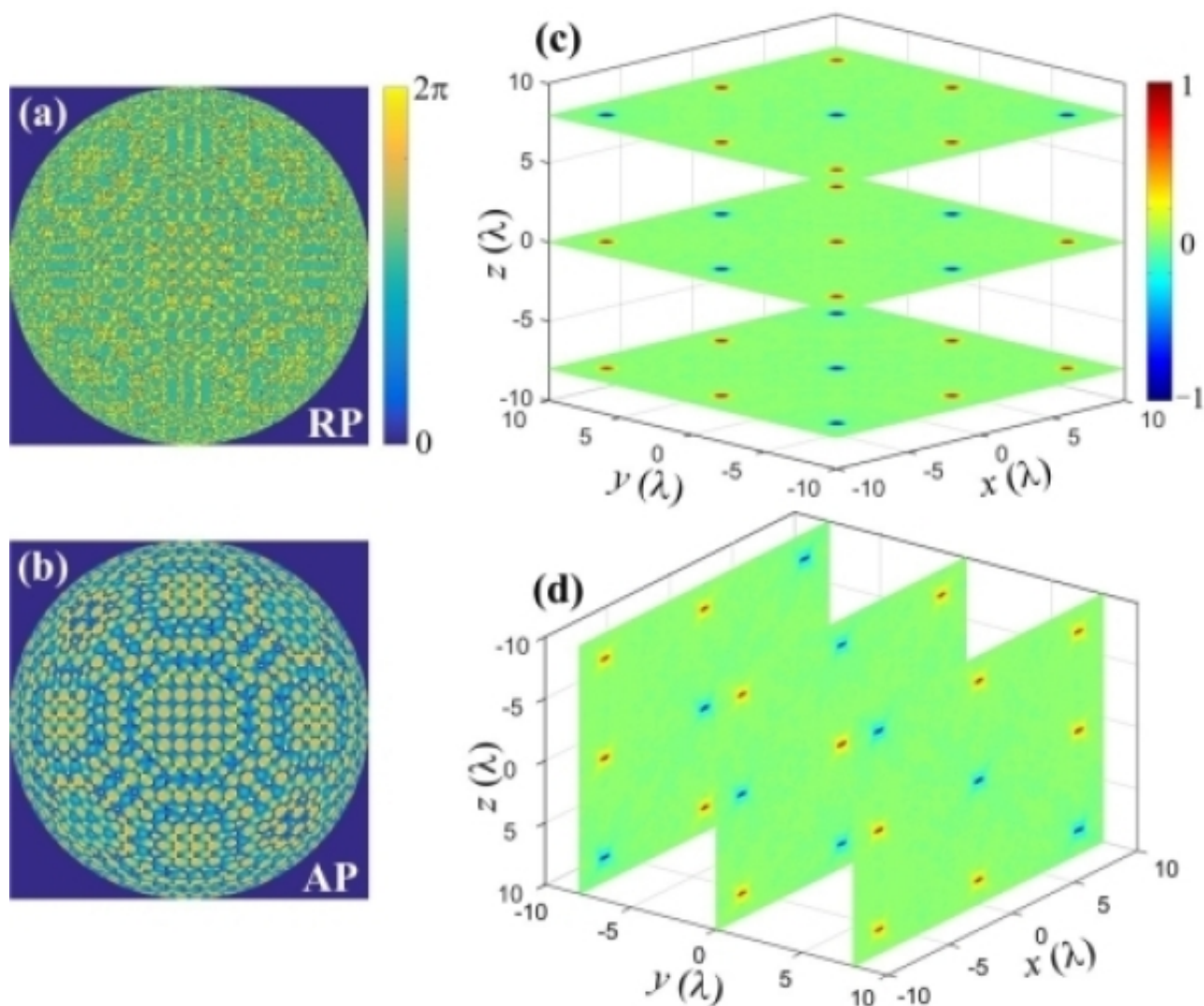
空间3D手性光场的产生。(a, b)加载在两个入射矢量光束上的相位分布, (c, d)横平面和轴平面的手性光场密度分布
