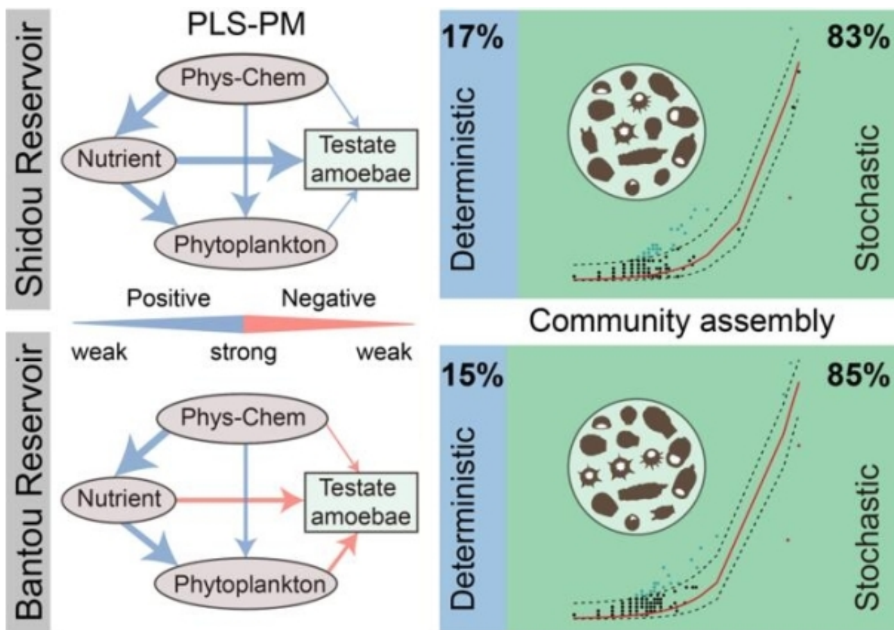
图2 论文摘要图
