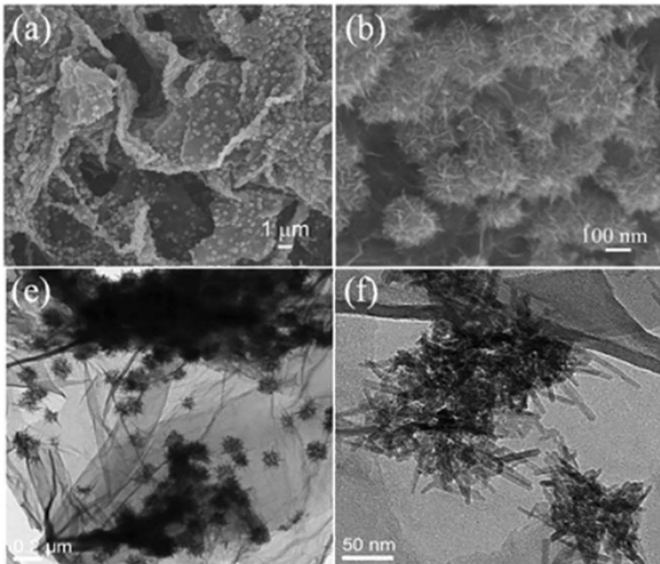
复合材料实例--石墨烯- 二氧化锰三维多孔复合材料 (a、b为扫描电镜图，e、f为复合材料的透射电镜图)
