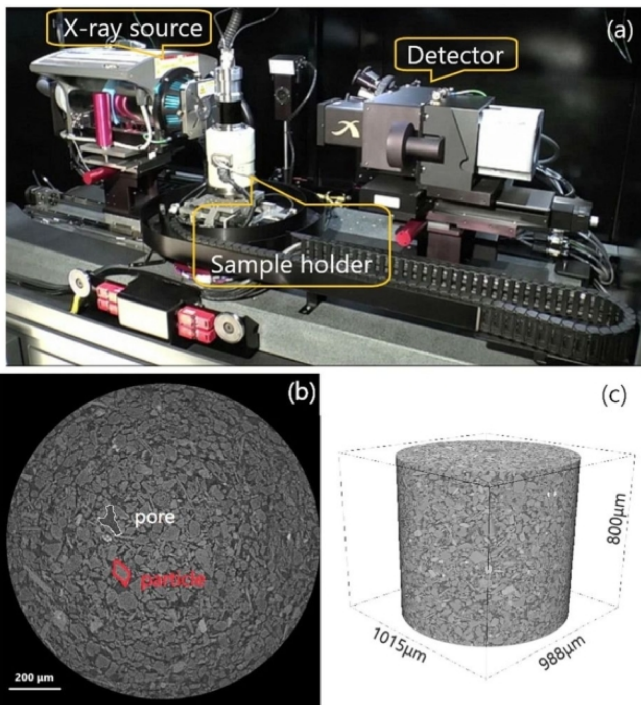
图1(a)微米CT设备；(b)1 μm分辨率二维灰度图；(c)重建后的三维结构体
