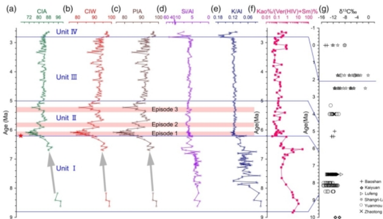
图2.昭通盆地古气候指标随年代的变化：硅酸盐风化指标 (a, b, c)；Si/Al和K/Al比值 (d, e)；粘土矿物比值 (f)。灰色箭头表示硅酸盐风化指数的变化趋势，红色五角星对应昭通古猿化石年代
