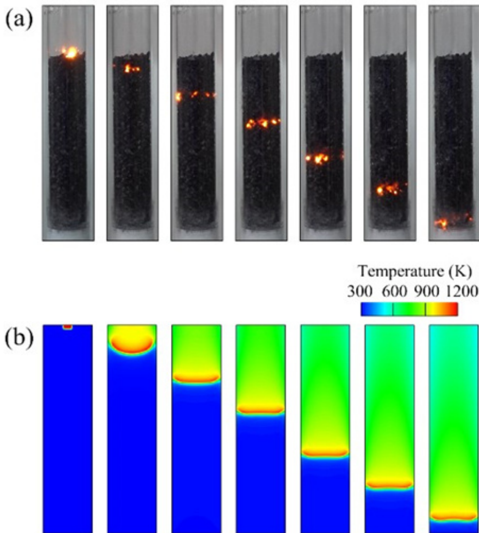
炽燃锋面的蔓延：(a) 实验现象、(b) 模拟结果
