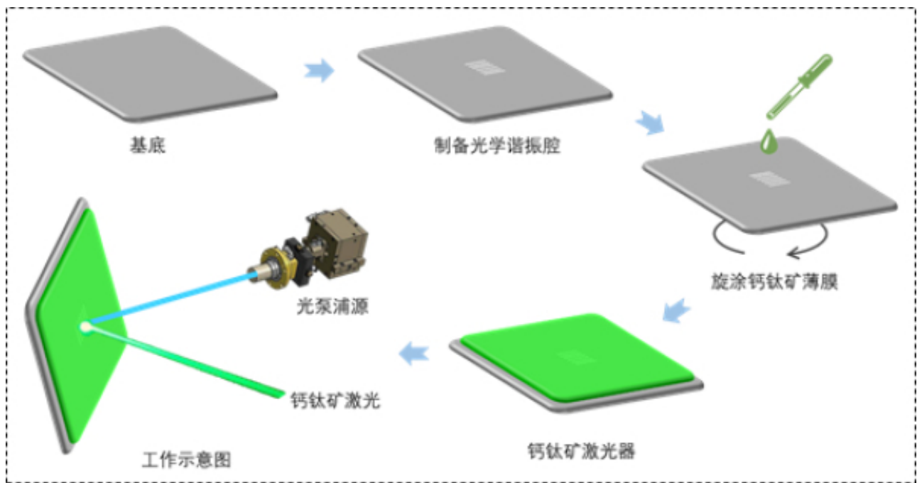
溶液旋涂制备低成本钙钛矿半导体激光器过程及工作示意图
