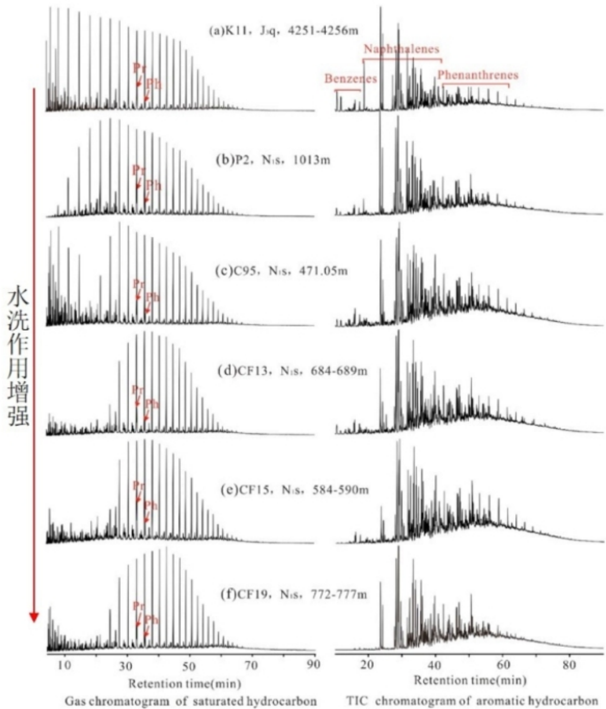
图2 原油中饱和烃和芳烃色谱图随着水洗作用的变化情况
