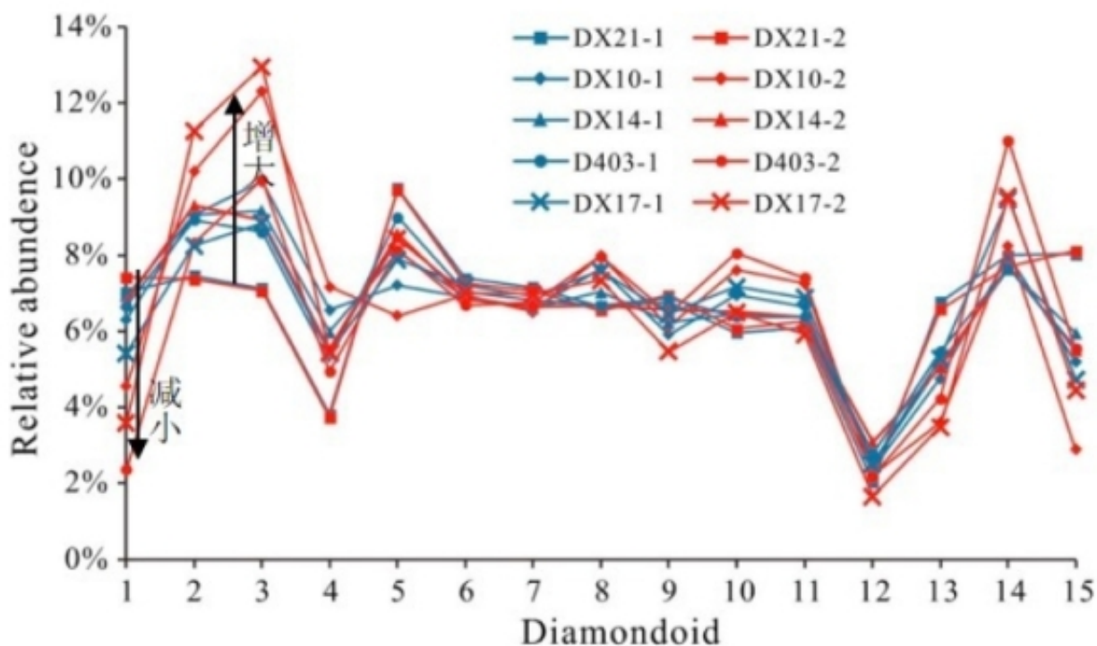
图3 原油中不同类型金刚烷相对含量受气洗作用的变化情况
