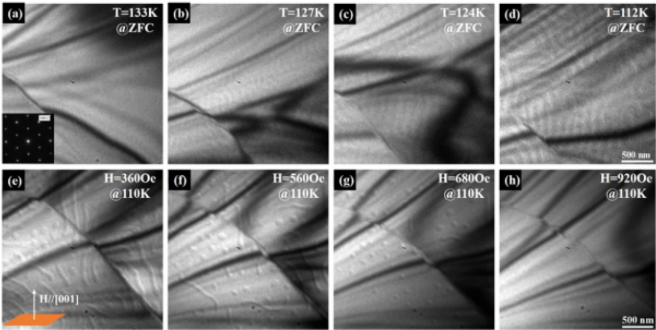
图2. (a-d) 冷操作后，不同温度下磁畴的欠焦洛伦兹照片；(a) 中插图为选区电子衍射，表明样品表面为ab晶面。当温度低于130K，条状磁畴自发地出现，随着温度降低更加清晰可见；(e-f) 在110K时，条状磁畴随外加磁场演化的欠焦洛伦兹照片；(e) 插图为外加磁场方向，垂直于a b晶面。随着垂直磁场增加条状磁畴(e) 逐渐转变为磁性斯格明子(f-g)，并最终形成铁磁态(h)，比例尺为500nm。
