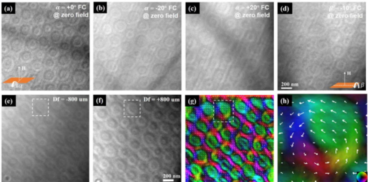
图3. (a-d) 倾角场冷(600Oe) 调控，温度在93K时磁性斯格明子的欠焦洛伦兹照片。【插图为倾角方向(a) \alpha = -20^\circ ，(b) \alpha = 0^\circ ，(c) \alpha = +20^\circ ，和(d) \alpha = -10^\circ 】。(e, f) 在93K、零场条件下拍摄的磁性斯格明子的欠焦和过焦洛伦兹图像。比例尺为200nm。(g) 结合(e)和(f)图，TIE处理之后的磁性斯格明子晶格面内自旋结构。(h) 单个磁性斯格明子面内自旋结构：各点磁化方向，如右下角色轮所示；磁性斯格明子的磁矩呈涡旋态排列，表明是布洛赫型磁性斯格明子。
