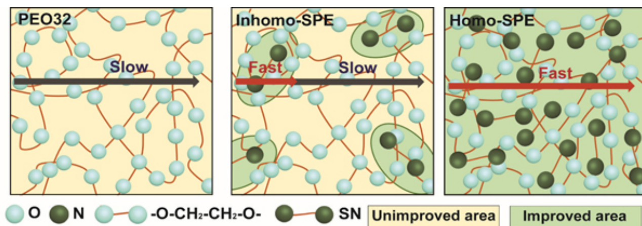
图2 固态电解质锂离子传输模式示意图
