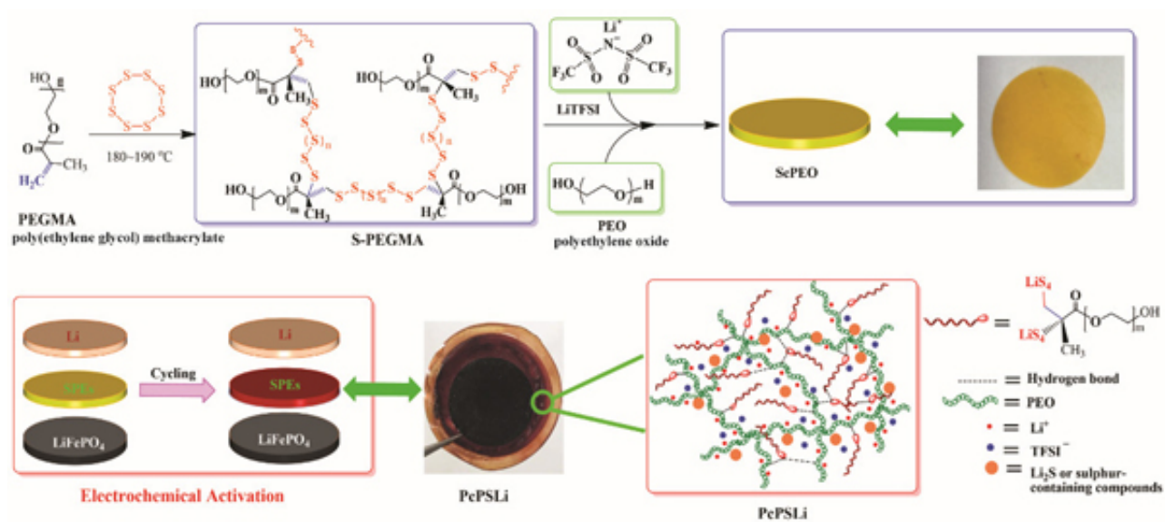
图1 多硫化锂接枝的固态电解质的制备过程
