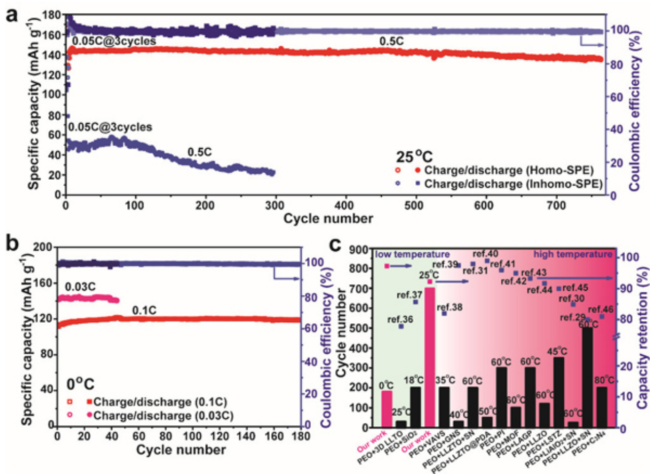
图4 固态电池性能
