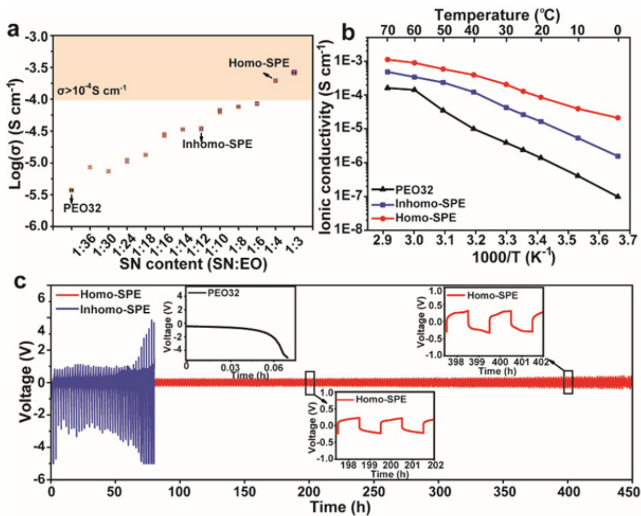
图3 固态电解质的电化学表征
