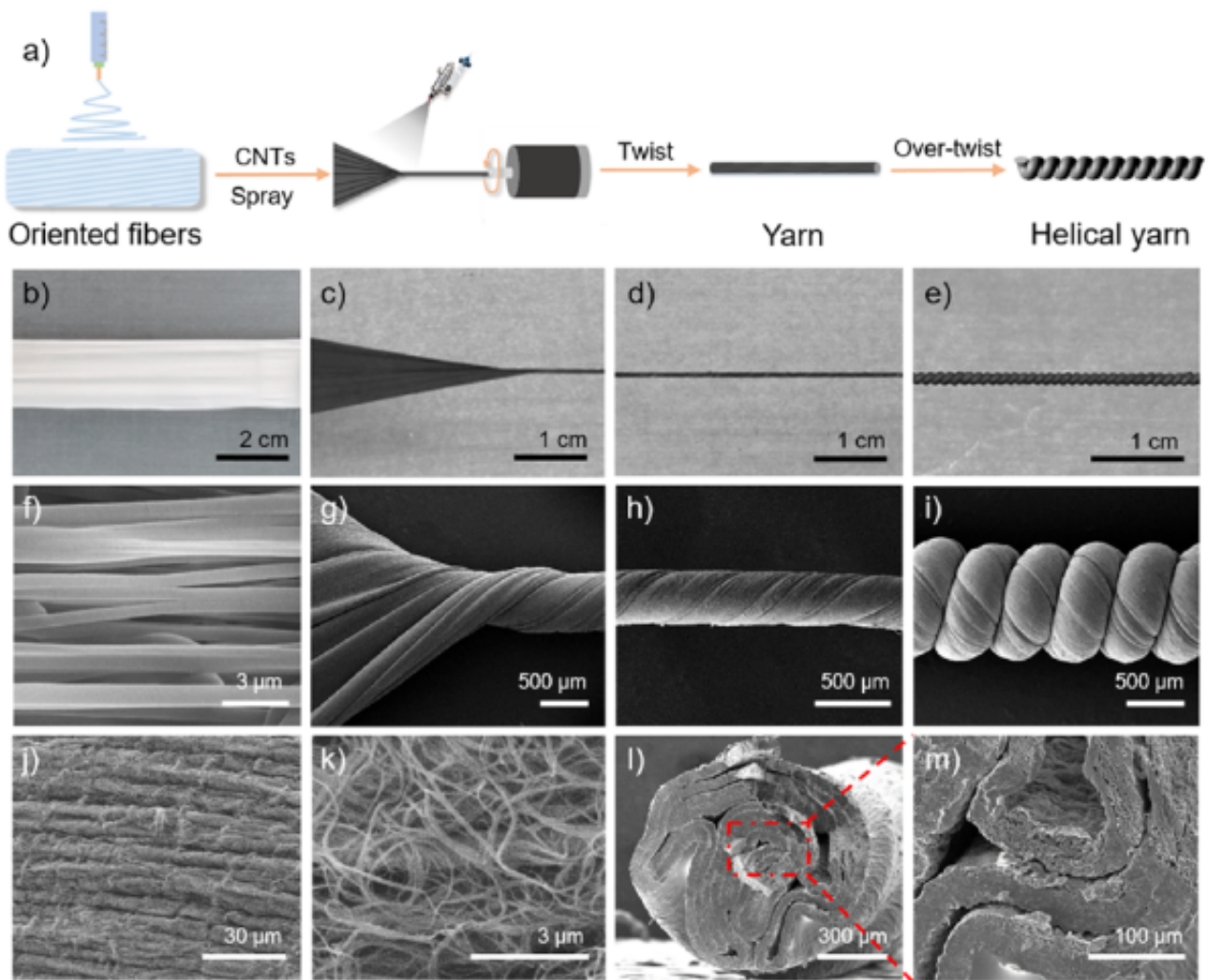
具有多尺度缠绕互锁螺旋结构的碳纳米管（CNTs）/聚氨酯（PU）纤维
