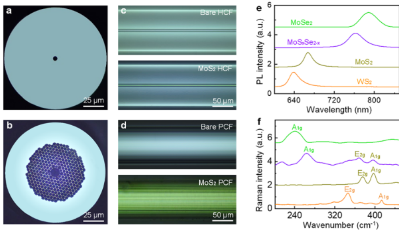
图2.制备不同结构二维材料复合光纤
