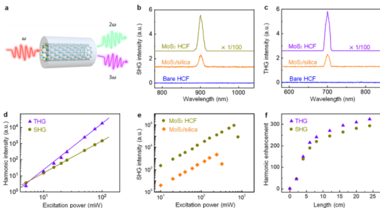
图3.二硫化钼复合光纤光频转化应用
