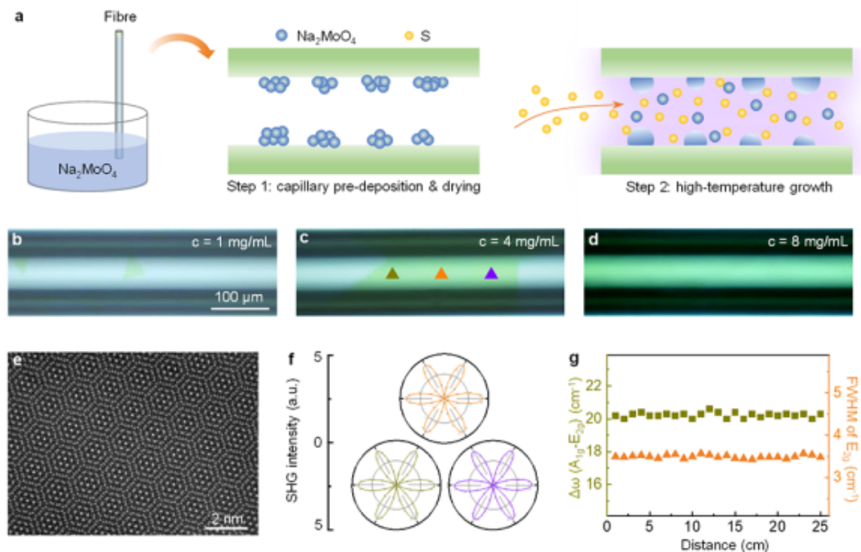
图1.两步化学气相沉积法制备MoS 2 复合光纤
