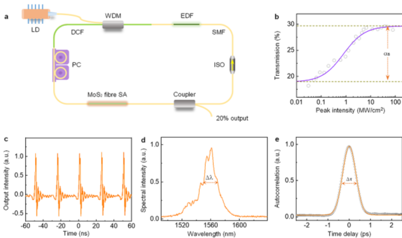
图4.全光纤超快锁模脉冲激光源应用
