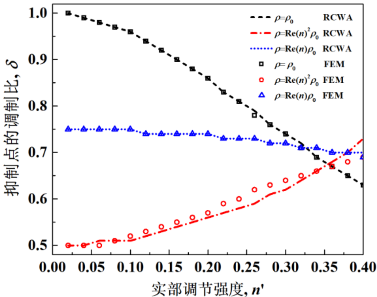
图3.不同调节方式下+1阶抑制点的调制比和实部折射率调节强度的变化关系（图/中科院声学所）
