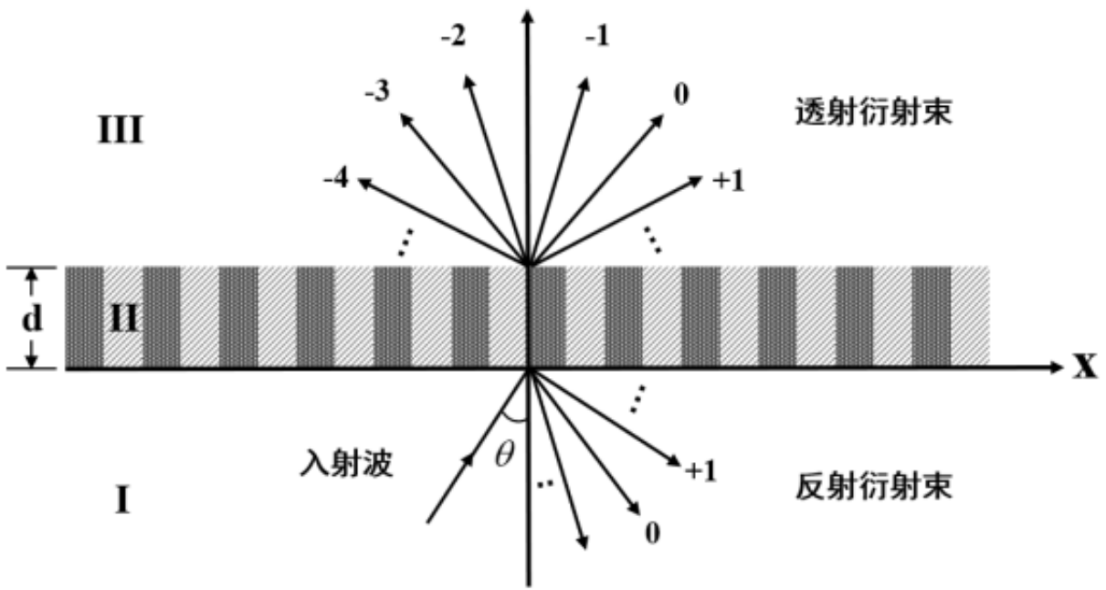
图1.声学衍射栅示意图 (图/中科院声学所)
