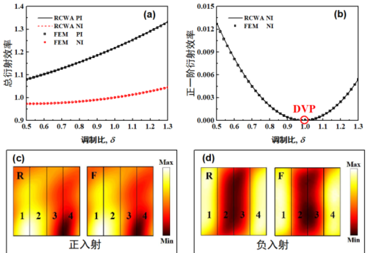
图2. (a) 总衍射效率 (b) +1阶衍射效率 (c) 正入射的声压分布 (d) 负入射的声压分布 (图/中科院声学所)
