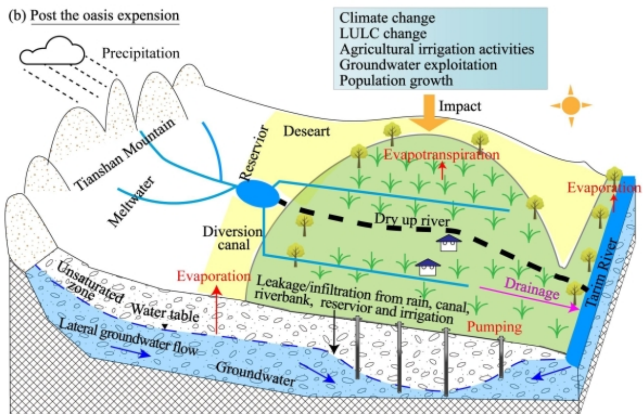
塔里木盆地典型绿洲扩张前后地下水循环过程概念图
