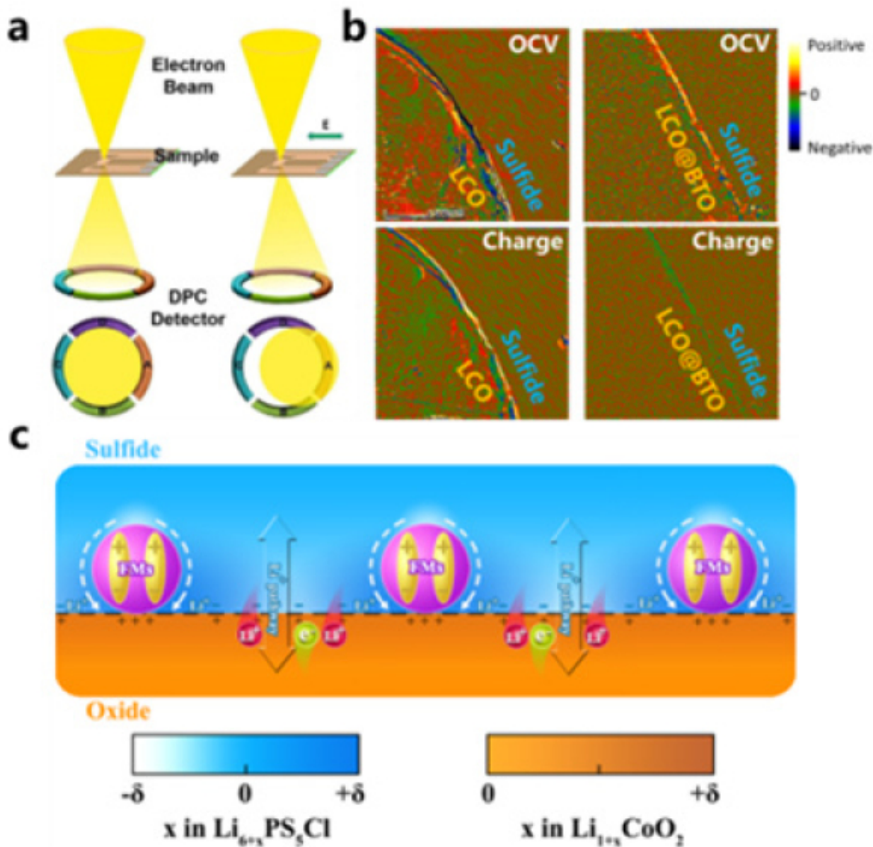
(a) 原位扫描透射电镜差分相衬成像技术工作原理示意图；(b) 钴酸锂/硫化物固态电解质界面锂传输行为的原位扫描透射电镜差分相衬成像结果；(c) 内建电场和化学势耦合技术改善界面锂传输机制示意图
