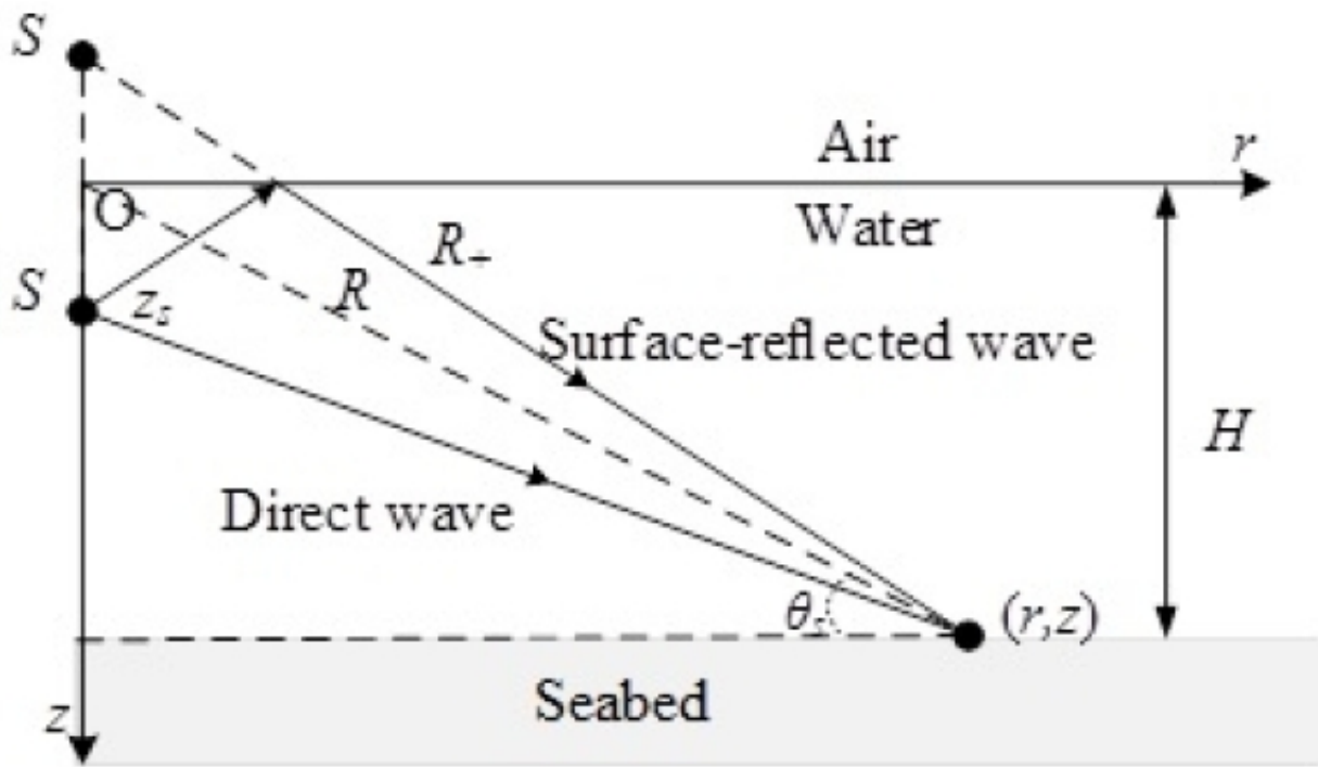
图1.深海大深度接收环境下直达波和海面反射波到达结构示意图（图/中科院声学所）
