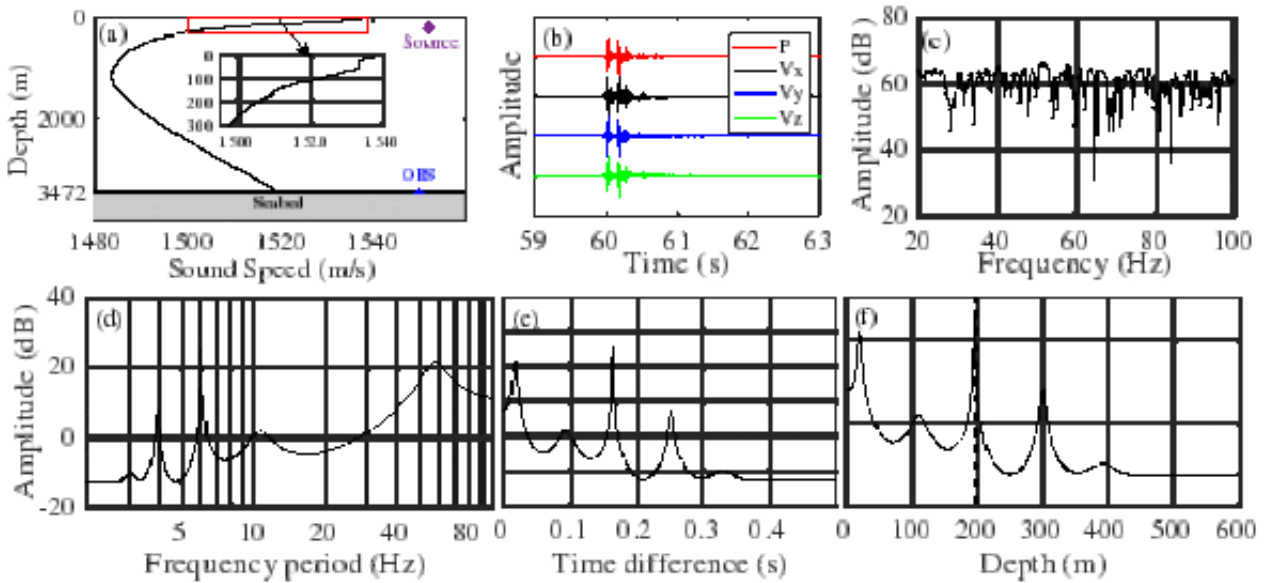
图2.收发距离为4.21 km的信号处理结果。（a）海水声速剖面及收发态势图；（b）声压和质点振速信号波形；（c）声强频谱；（d）-（f）为MUSIC处理后的声强频谱结果，对应X轴分别为频率干涉周期、到达时延差和声源深度（图/中科院声学所）
