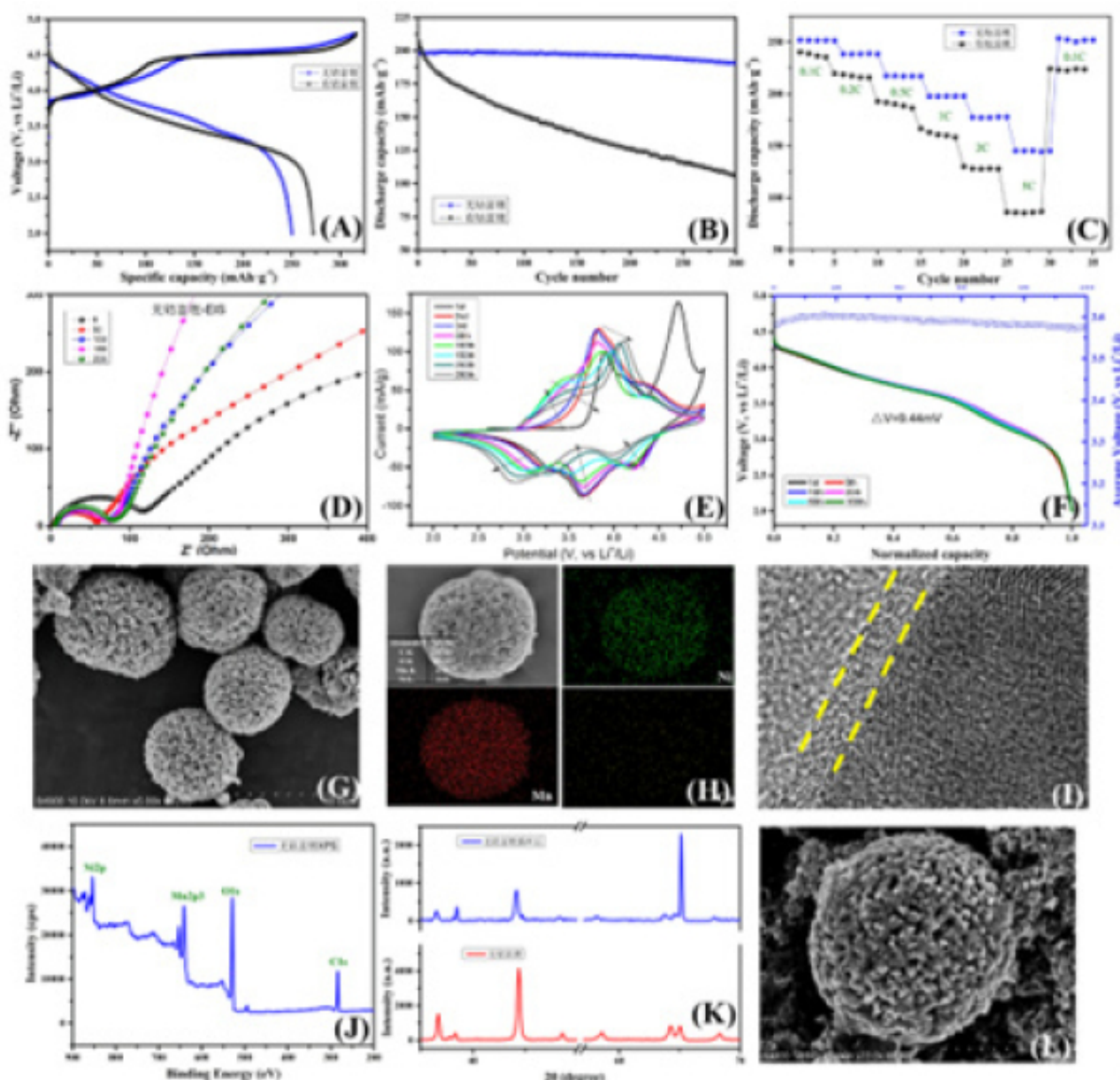
无钴富锂锰基正极材料体系的电化学性能 (A-F) 和相关结构表征 (G-L)
