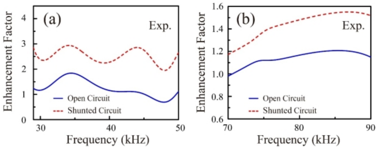
图2.可调式声学阻抗匹配层在插入钢/有机玻璃（左图）和钢/铝后的声能透射增强因子（右图）
