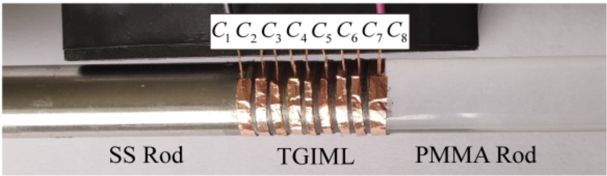
图1.基于压电分流电路的可调式声学阻抗匹配层
