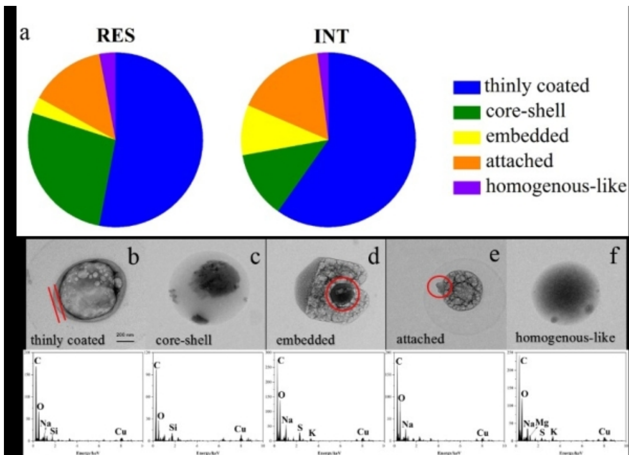
图1.云滴残留颗粒（RES）和间隙颗粒（INT）中有机物颗粒的混合结构及其占比
