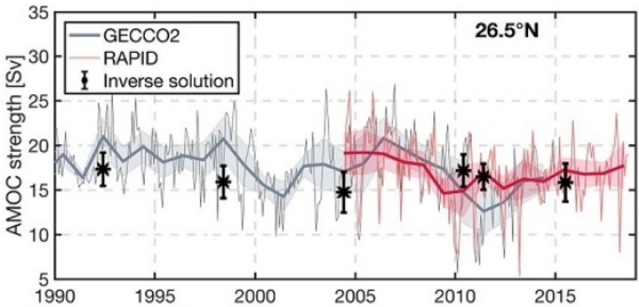
图3.北大西洋AMOC强度时间序列
