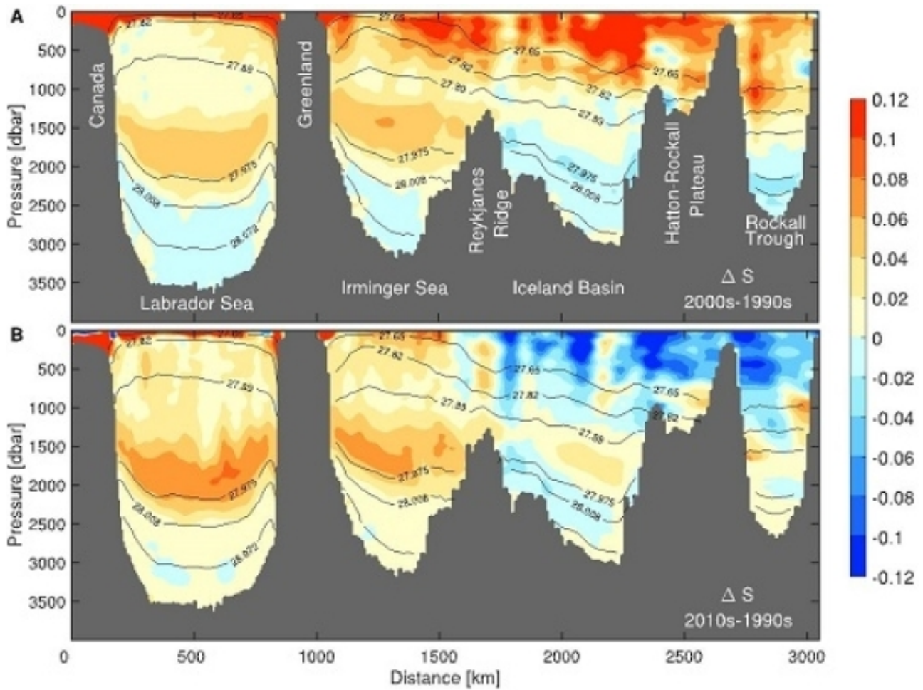
图2.副极地北大西洋盐度的年代际改变
