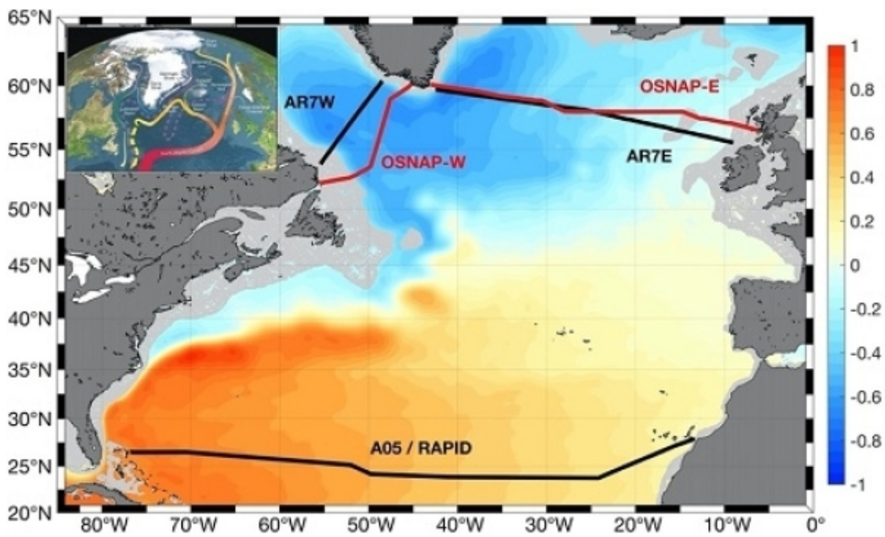
图1.北大西洋地图及大西洋翻转流示意图
