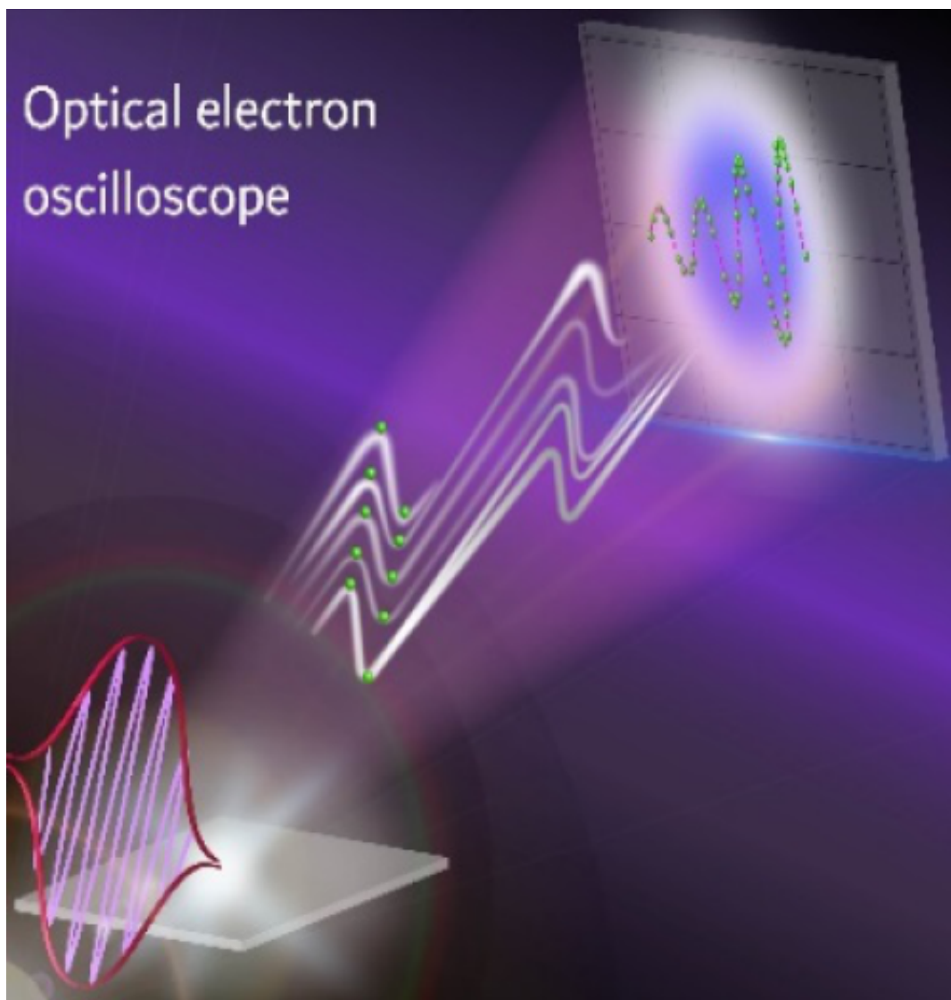
图3. “全光阿秒电子示波器”概念图 图2展示了不同空间分布电子在光场相位下分布及空间分布。周期性发射的阿秒电子脉冲在激光场调制下形成了条纹结构分布，这一作用过程把电子按时间的先后顺序转换成了空间投影，根据电子空间分布可直接反演其阿秒时间动力学过程。“全光阿秒电子示波器”概念（图3）中“偏压”电场场强 10^{12}
