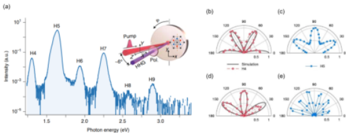
(a) 拓扑绝缘体产生高次谐波实验布局与光谱图。(b) - (c) 平行驱动光偏振方向的 (b) 4 级次, (c) 5 级次谐波强度的角度分布。(d)、(e) 对应 (b)、(c), 为垂直分量的角度分布 研究团队单位: 上海光学精密机械研究所
