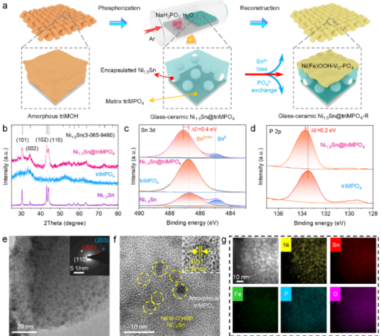
图2.通过低温磷化方法合成了具有双相结构的微晶玻璃，结合XRD、XPS、HRTEM、EDS-Mapping等技术，证明其中结晶相是 \text{Ni}_{1.5}\text{Sn} 纳米颗粒，非晶相是 \text{triMPO}_4 三金属磷酸盐
