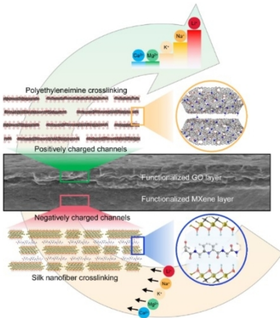
基于仿生纳米通道膜的离子筛分
