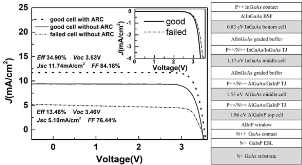
图1.IMM四结太阳能电池J-V曲线和结构示意图
