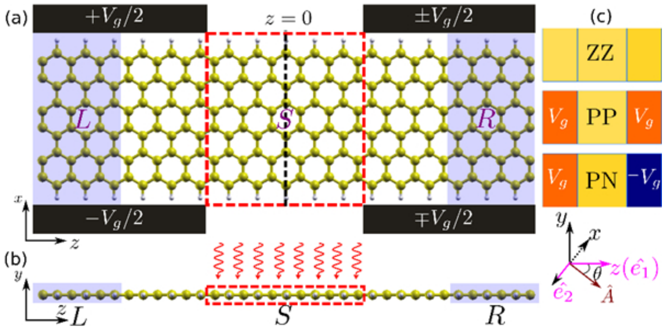
图1.基于带宽为6的锯齿形石墨烯纳米带构建的自旋光电器件 (a-b) 以及 (c) 器件的三种栅压构型
