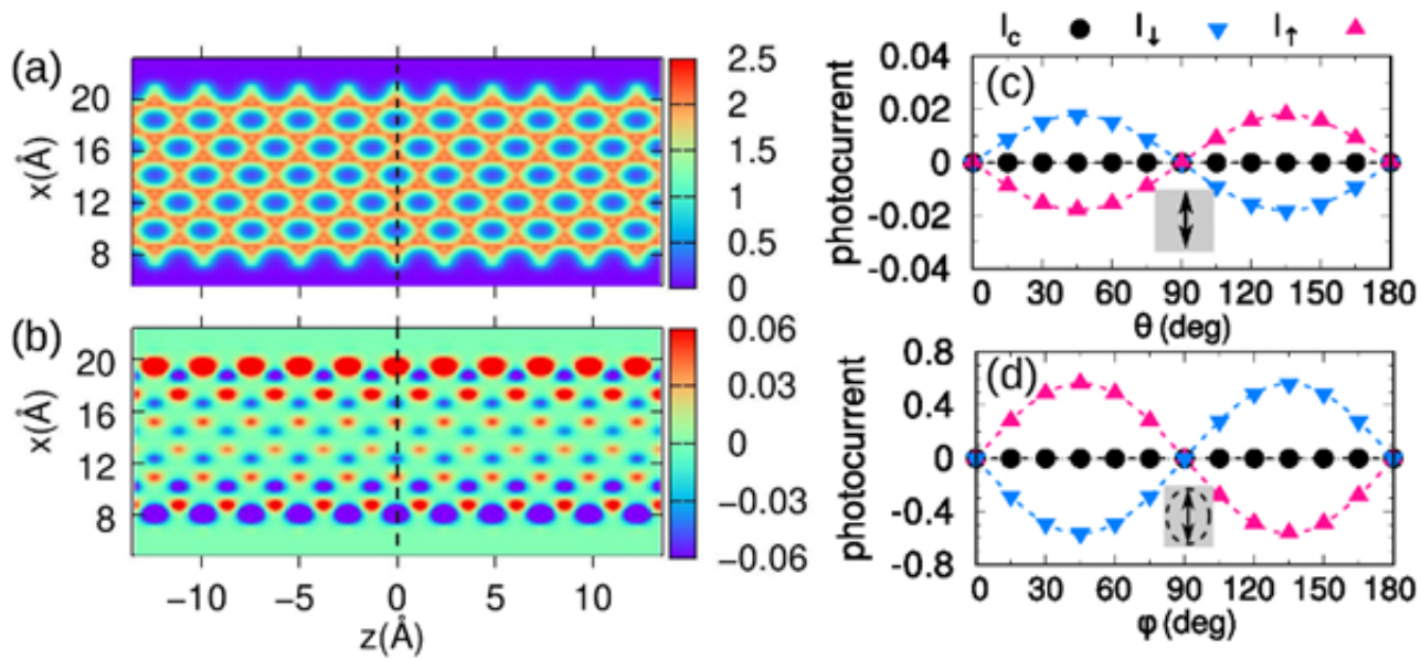
图3.锯齿形石墨烯纳米带体系的纯自旋流产生示意图
