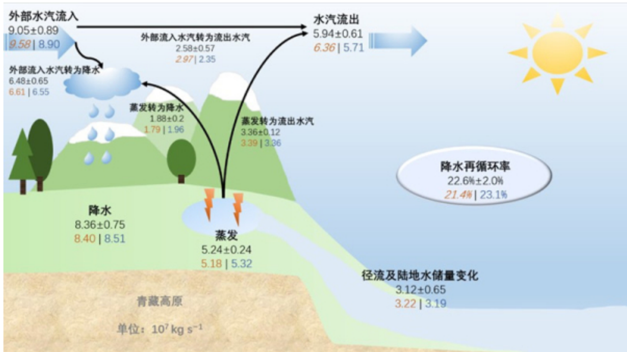
青藏高原夏季大气水循环示意图。黑色数字表示气候态及年际变率，红色（蓝色）数字表示前冬发生厄尔尼诺（拉尼娜）事件，斜体表示变化通过了 p=0.1 的双边Students' t检验 研究团队单位：大气物理研究所
