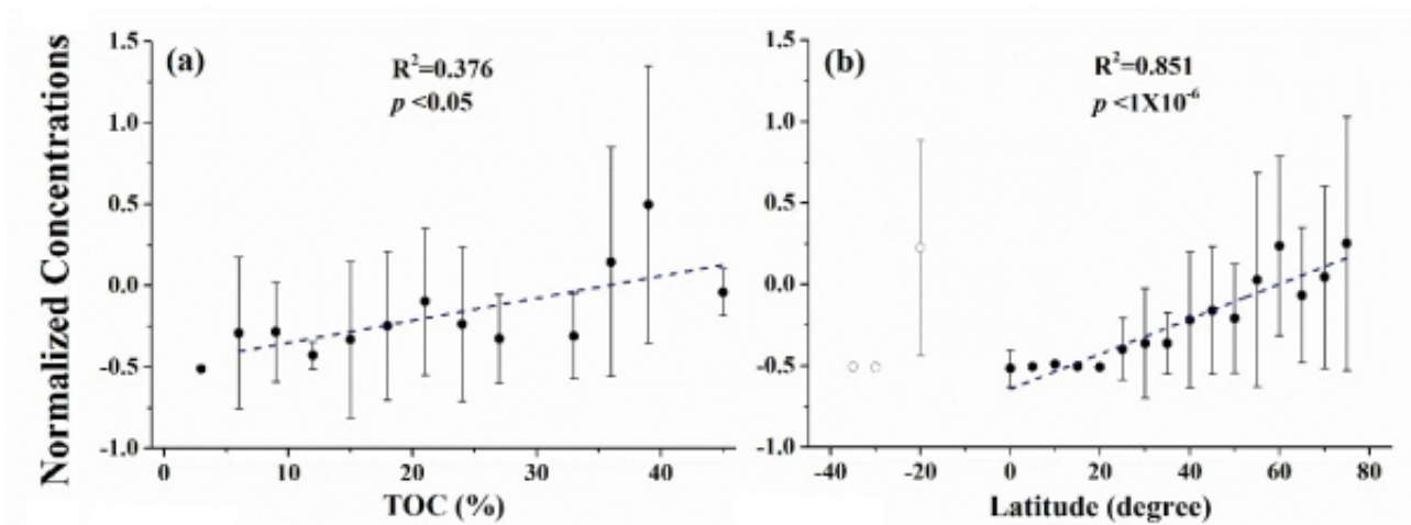
图2 土壤有机碳（TOC）和纬度对森林土壤POPs分布的影响 研究团队单位：青藏高原研究所
