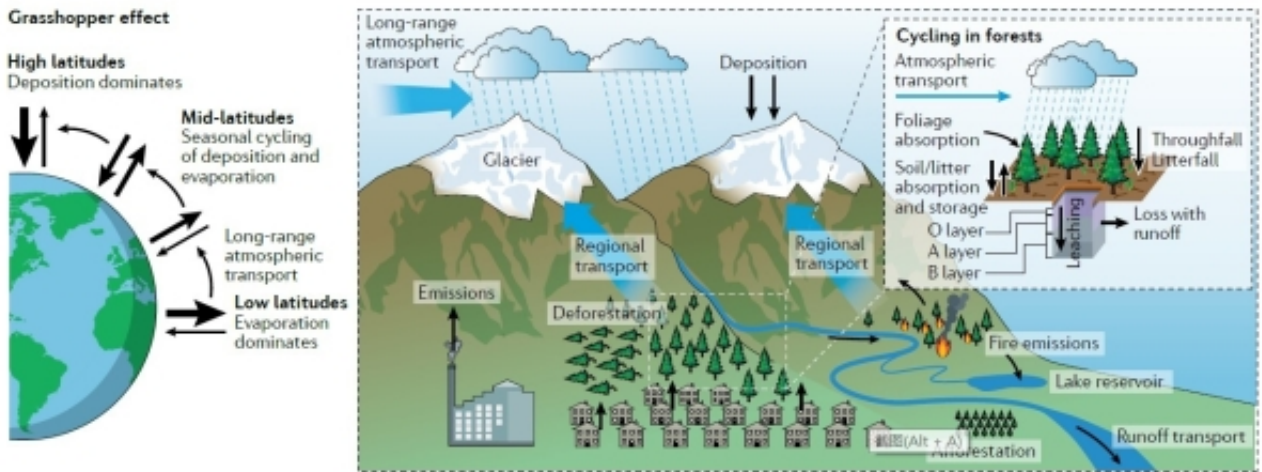
图1 POPs全球迁移模式（左图）及森林中POPs的循环过程（右图）
