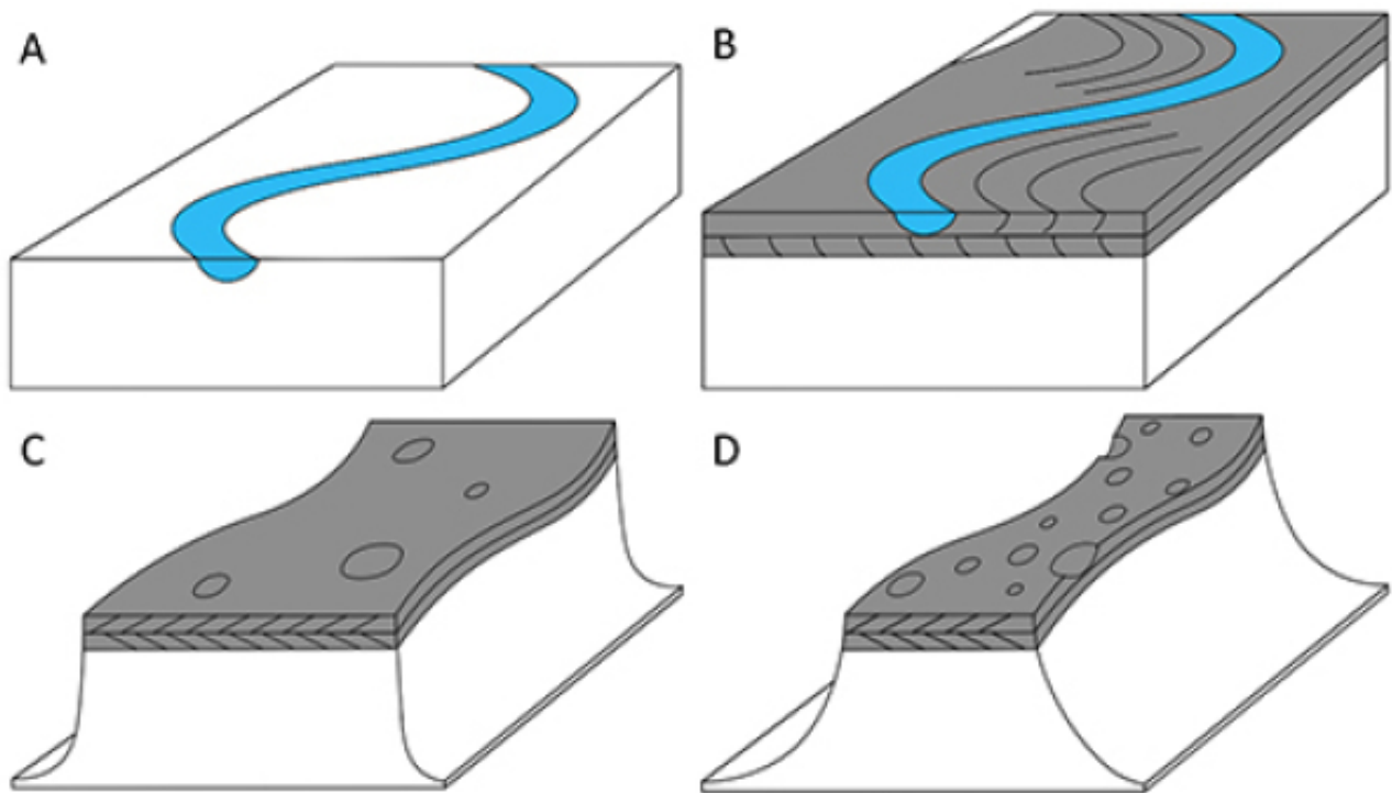
图3. (a) 一条活跃的河流流经火星表面。(b) 洪泛平原形成沉积，物质开始迁移。(c) 河道带开始被侵蚀挖掘（黑色圆圈代表撞击坑），原始河道消失。(d) 在后期长时间的风化侵蚀作用下，河道带形成了宽度不定的脊状地貌。
