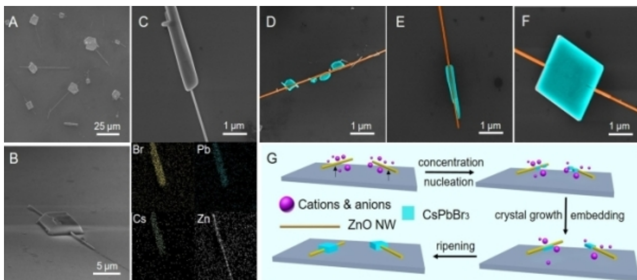
CsPbBr 3 -ZnO异质结的生长机理与形貌表征图
