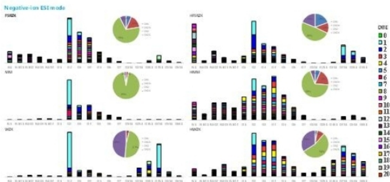
三种烃源岩游离沥青和结合沥青中杂原子化合物的组成分布图（负离子FT-ICR MS）
