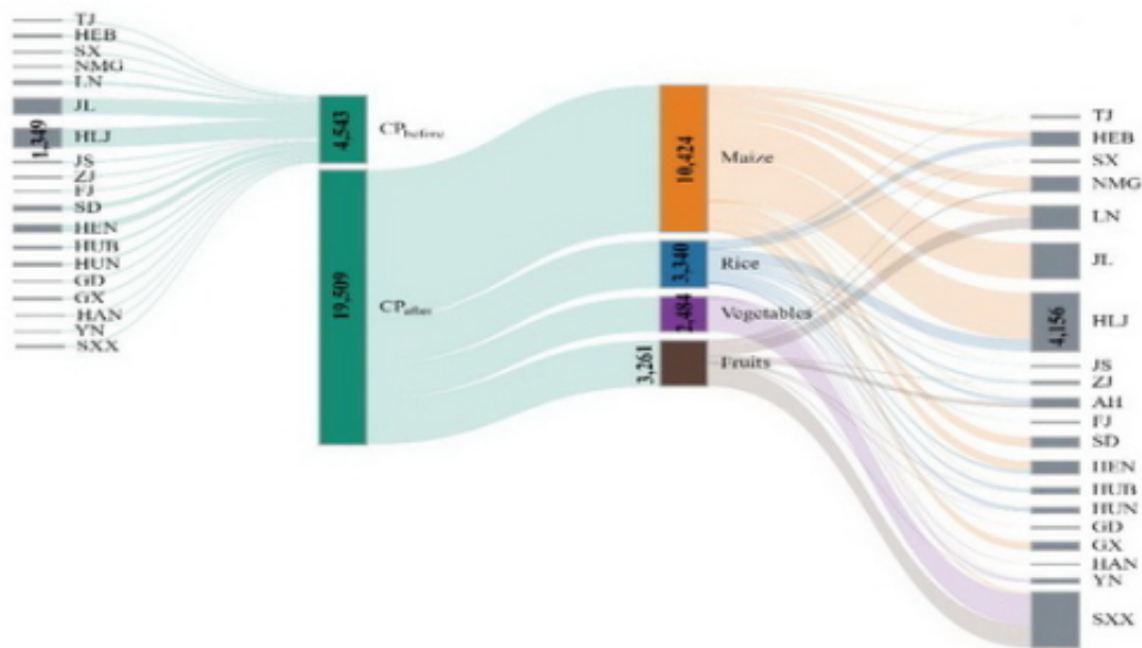
图3.大豆进口导致的种植结构转变对施氮量 (NA, 10^3 ton) 的影响
