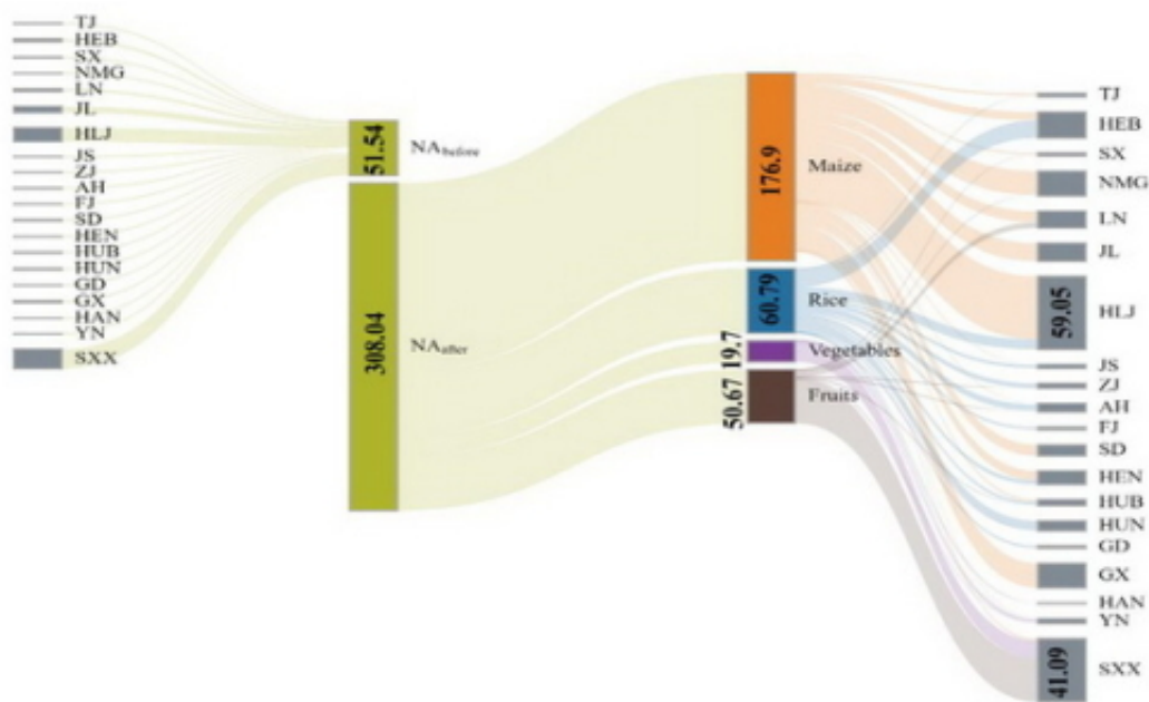
图1.大豆进口导致的种植结构转变对作物产量 (CP, 10^3 ton)
