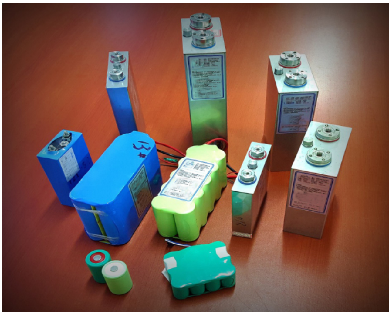
图2.各种型号的宽温镍氢电池产品
