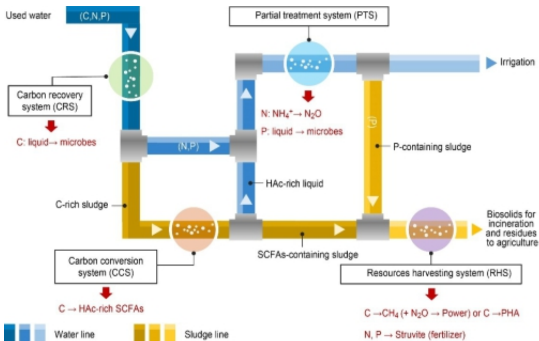
图1.REPURE范式图示。污水有机物在碳源捕获系统(CRS)中得到富集后进入碳基转化系统(CCS)制备以乙酸为主的短链脂肪酸;转化后的碳源一部分进入污水处理系统(PTS)供以生物脱氮除磷。PTS系统制备的再生水用于土地浇灌,而PTS和CCS系统产生的生物污泥则进入资源回收系统(HRS)进行资源转化。大部分有机质在此转化为甲烷( \text{CH}_4 ),其余则供以合成聚合物(PHA)。污水氮元素大部分在PTS系统中转化为氧化亚氮( \text{N}_2\text{O} )并与 \text{CH}_4 进行共燃烧产能,磷元素则以鸟粪石(Struvite)形式进行缓释肥制备。剩余污泥经焚烧发电后进行营养元素的土地利用。土壤生态系统将协同转化生物分解代谢产物二氧化碳,并促进营养元素的末端利用。
