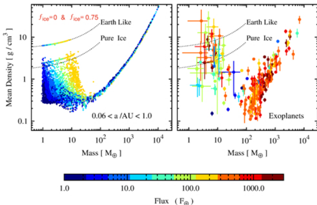
图1.模型得到的行星族群(左)和系外行星(右)在质量-平均密度图上的分布。该结果验证了模型所依赖的行星形成和演化理论。
