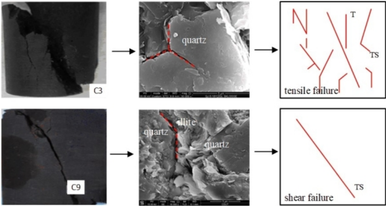
图3.页岩高应力条件下破裂机制
