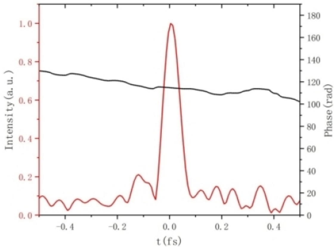
阿秒脉冲时域及相位分布
