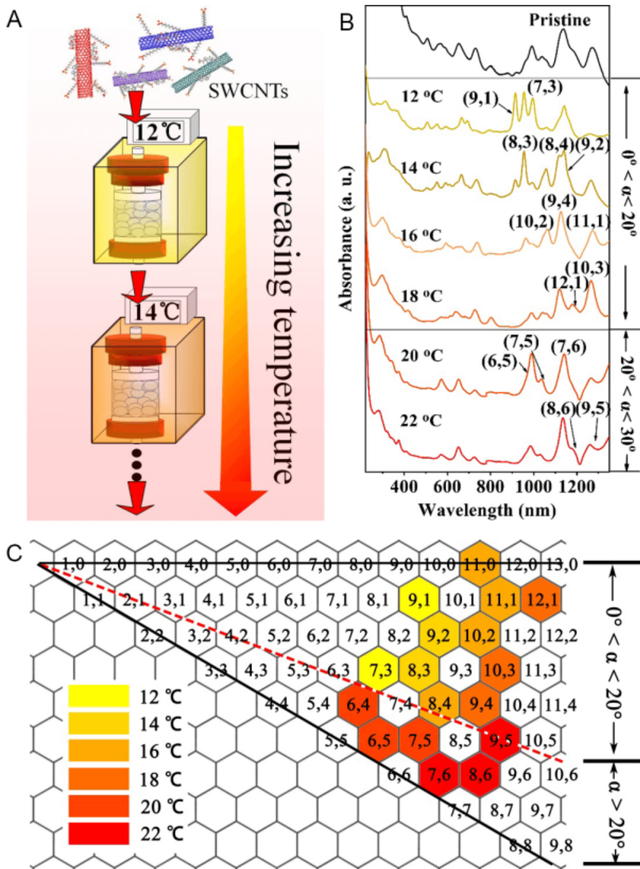
图1.温度调控实现碳纳米管手性角的选择性吸附。A、分离碳纳米管手性角示意图；B、十二烷基
