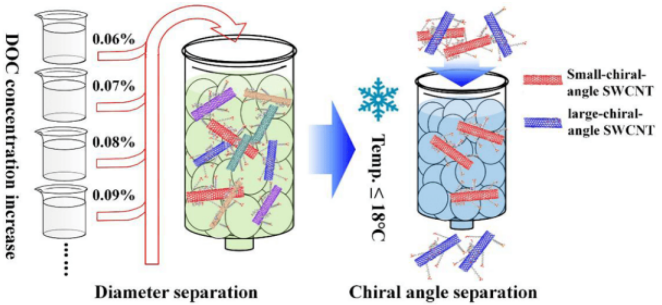
图2.通过直径、手性角连续分离单一手性锯齿型和近锯齿型碳纳米管示意图
