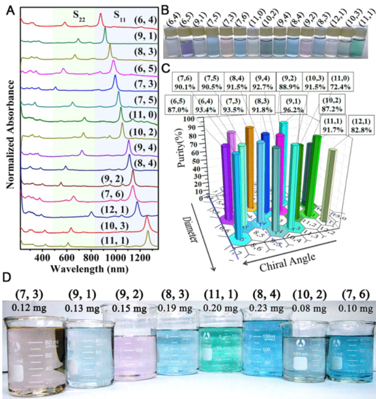
图3.分离制备的单一手性碳纳米管表征。A、分离制备的15种单一手性碳纳米管光吸谱及B溶液照片；C、各种单一手性碳纳米管的纯度分布；D、次毫克量级单一手性碳纳米管溶液照片
