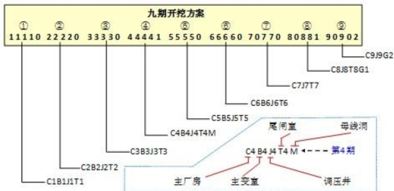
图1.洞群分层开挖方案组码与解码示意图
