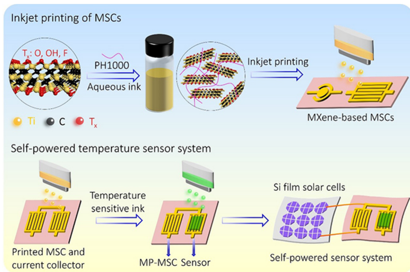
喷墨打印微型超级电容器及自供电集成系统构筑的示意图
