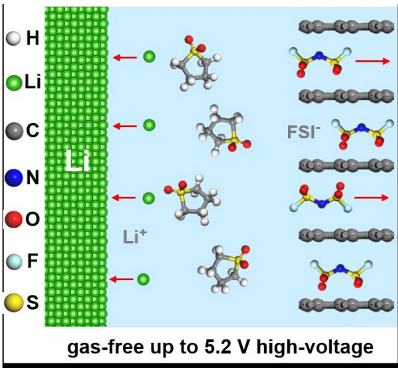
基于高电压浓缩电解液双离子电池的工作示意图
